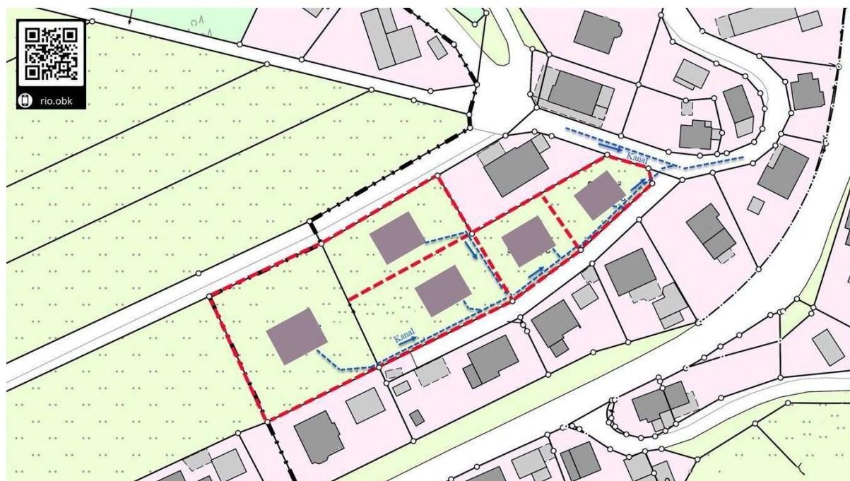
Konzept mit Teilung und Entwässerung
