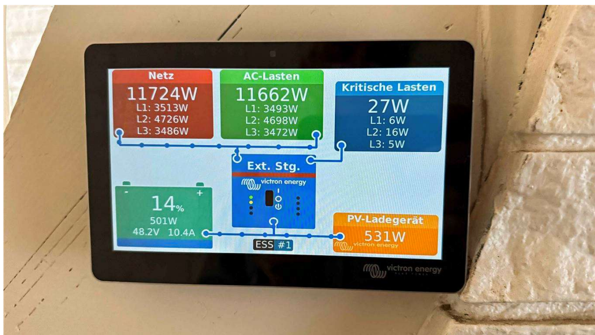
smarte Energieübersicht
